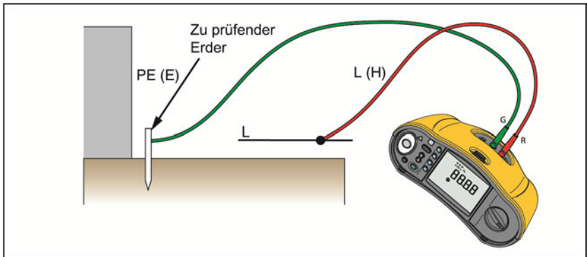
Abbildung 17. Zweikabelanschluss für Erdungswiderstandsschleifentest (Modus ohne RCD/FI)
