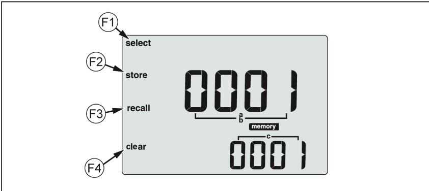
Abbildung 18. Speichermodus
